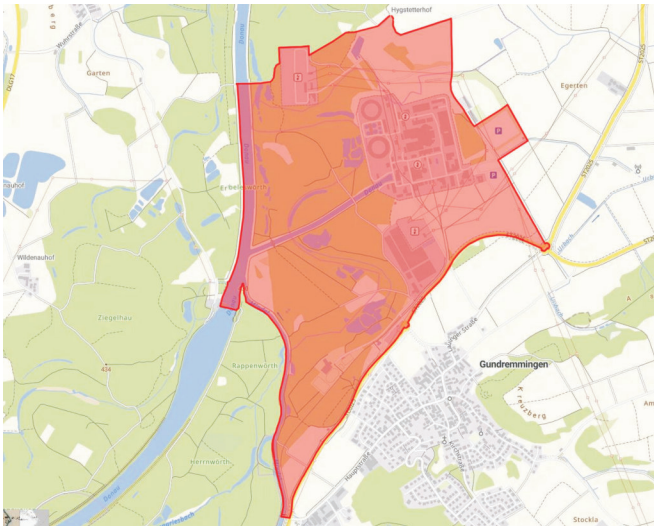
Abbildung: Absperrbereich zur Sprengung der Kühltürme des Kernkraftwerks Gundremmingen
