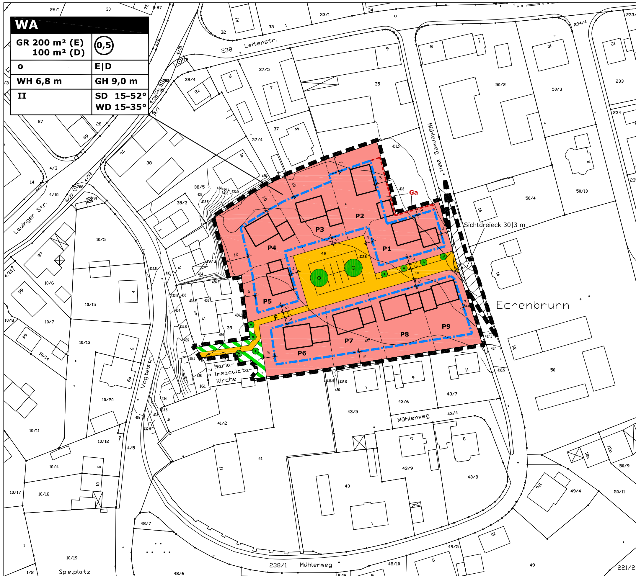
Planzeichnung Maßstab 1:1.000
